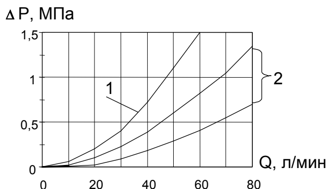
Рисунок 1 – График зависимости перепада давления от расхода гидрораспределителей типа РГС4-6/3СЕ
