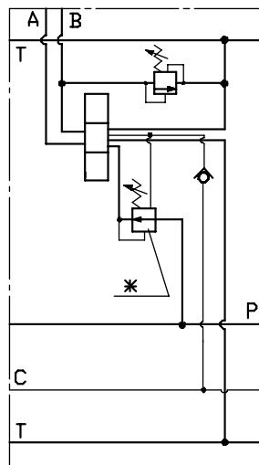
Исполнение 2— с предохранительным клапаном в гидролинии В
